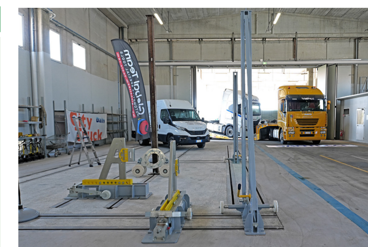
IMPONENTE Unica struttura coperta sul territorio con attrezzature dedicate, il Centro revisioni per veicoli pesanti, con all'interno un'ala dedicata alla carrozzeria pesante, si concretizza in un capannone di 2.500 metri quadrati e 3.500 mq di piazzali esterni.
